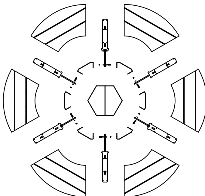
3. Bovenaanzicht tafelconstructie met alle onderdelen. Bouten aan de binnenkant van de verbindingspanelen.
