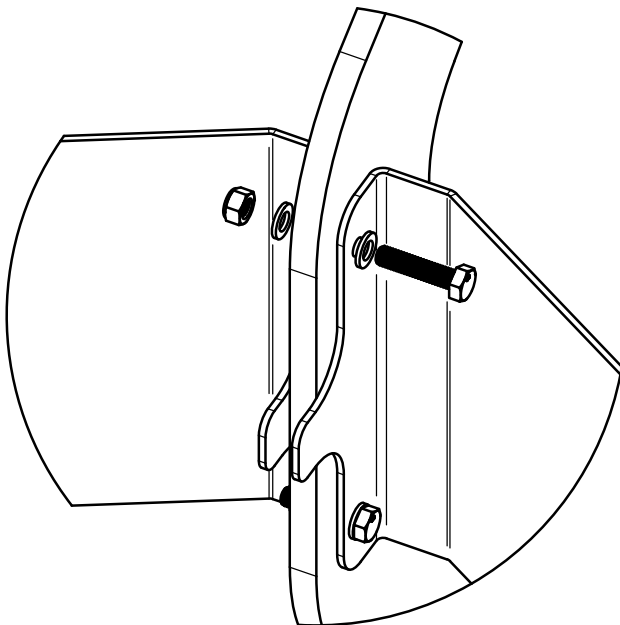
4. Maak 2 verbindingsplaten vast aan een poot.
