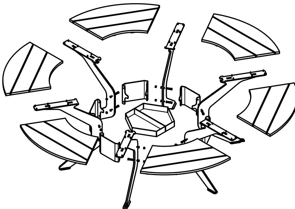
1. Alle onderdelen van de tafelconstructie.
